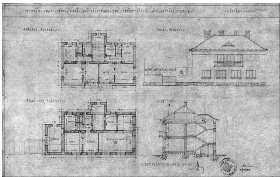
A szolgálati lakás korabeli tervrajza
